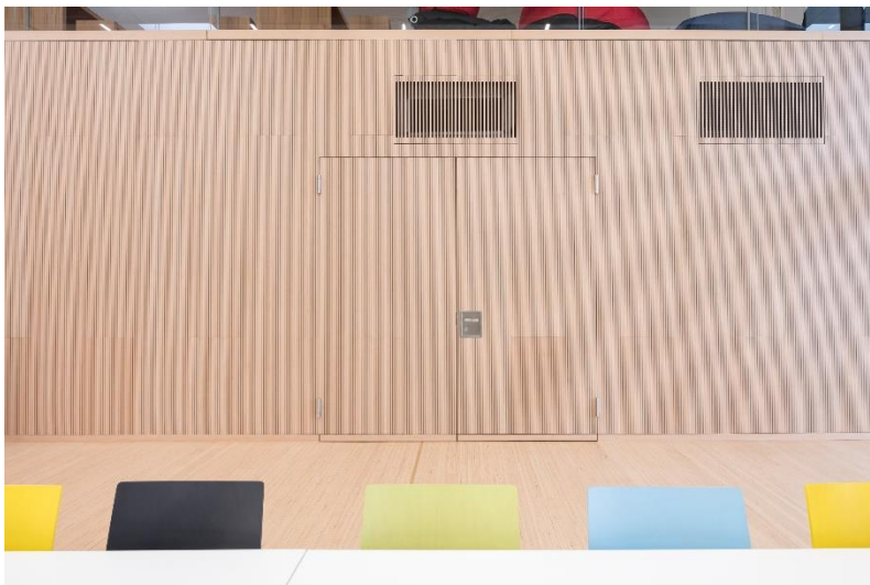
Bild 7: Die zweiflügelige Schörghuber Tür ist wie die umliegenden Wände mit Buchenfurnier beplankt und integriert sich flächenbündig und somit nahezu unsichtbar in den Raum.
