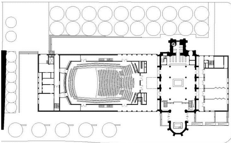
Bild 10: Grundriss Erdgeschoss des Neu- und Bestandbaus.
