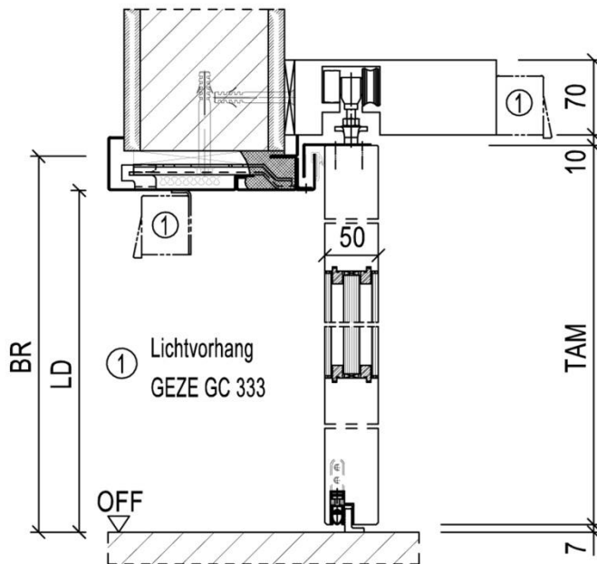
Bild 3: Zeichnung der einflügeligen Brandschutz-Schiebetür Typ 3N-ST in Mauerwerk. Zweiteilige Schiebetürstahlzarge, Automatik-Ausführung, auch mechanisch erhältlich.
