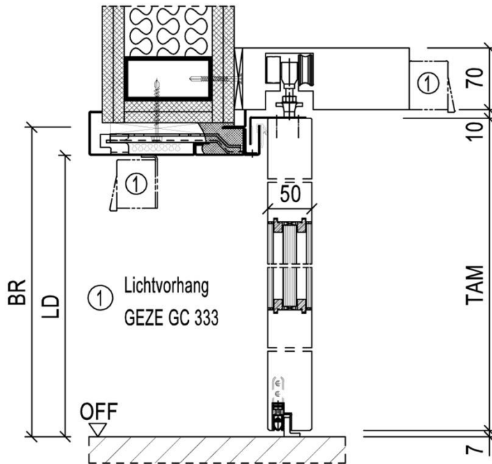
Bild 5: Zwei-schalige Stahlzarge zur Abdichtung mit Fugenfüller für den Einbau der Brandschutz-Schiebetüren in Leichtbauwände.
