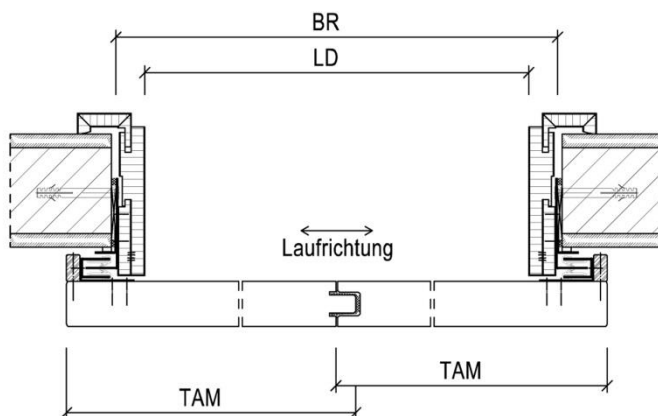
Bild 4: Zeichnung der zweiflügeligen Brandschutz-Schiebetür Typ 4N-ST in Mauerwerk mit dreiteiliger Holzfutzarge.
