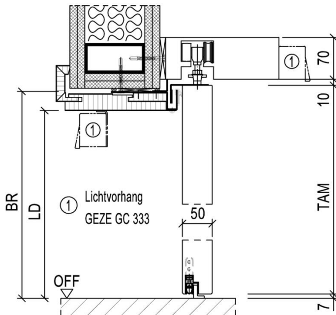
Bild 6: Drei-schalige Holzzarge zur Hinterfüllung mit PU-Schaum oder Mineralwolle für den mörtelfreien Einbau der Brandschutz-Schiebetüren.
